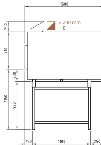
RIGHT ELEVATION
